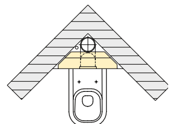
Einbaubeispiel: WC-Stein 110 cm, abgeschrägt; Befestigung in einer Ecke mit Falleitung
