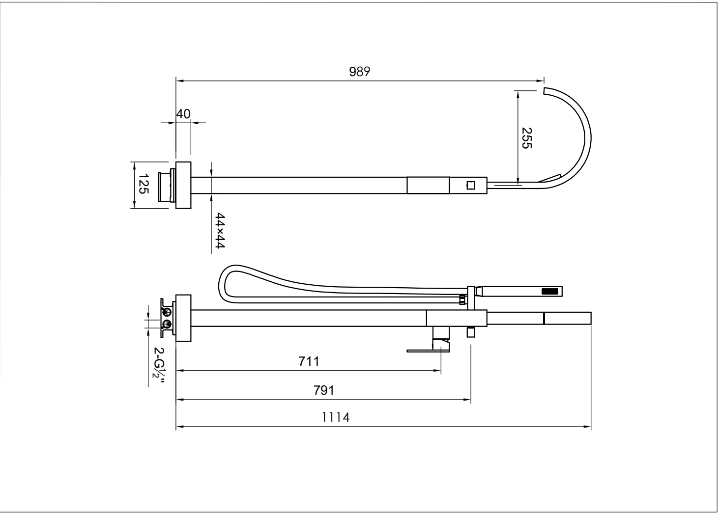
Technische Zeichnung
