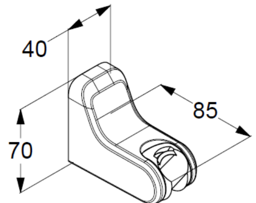
Maßzeichnung
