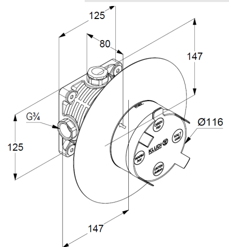
Maßzeichnung
