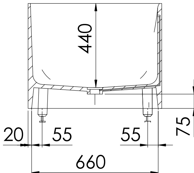
SCHNITT B-B
