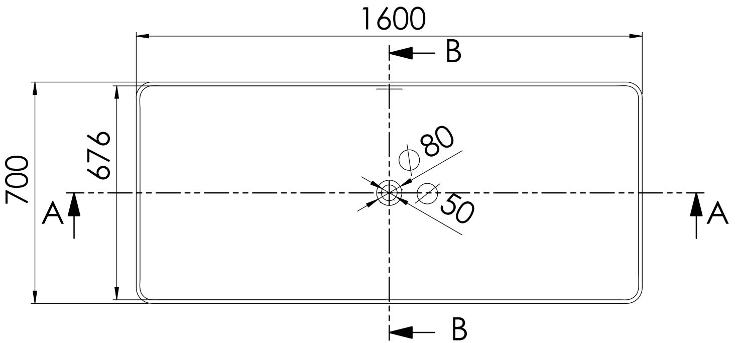
SCHNITT A-A
