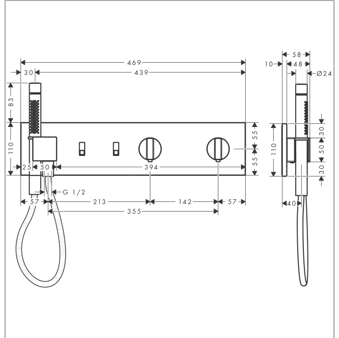
Maßzeichnung
